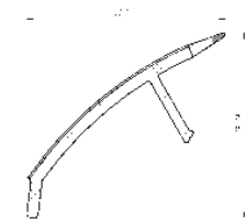
FINO Nischenrückwand-Kombiprofil Unterprofil – zur Montage der Nischen- rückwand auf der Arbeitsplatte
